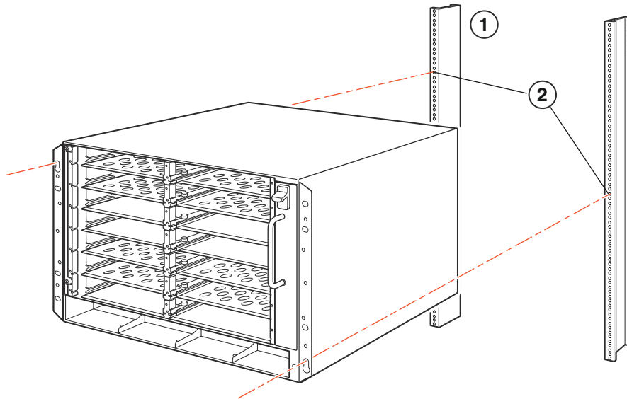
1 Geräte-Rack 2 Montagelöcher
